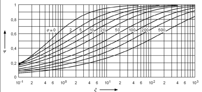
Figura 7 - Factor \psi para la fuerza de tracción en conductores flexibles
