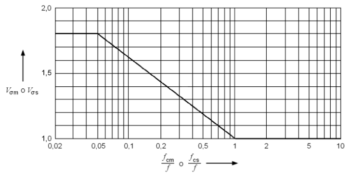
Figura 5 - Factores V_{rm} y V_{rs} a utilizar en el caso de recierre automático trifásico
